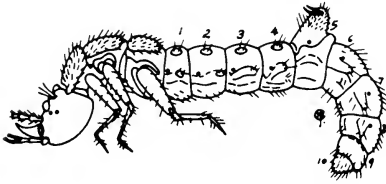
Fig. 174. Megacephala carolina (L.).
